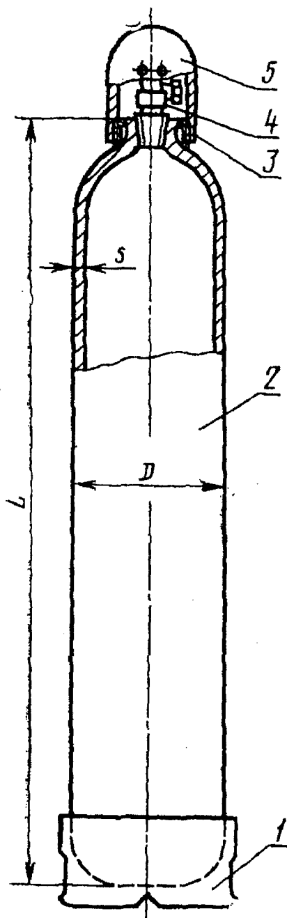
Горловина баллона
